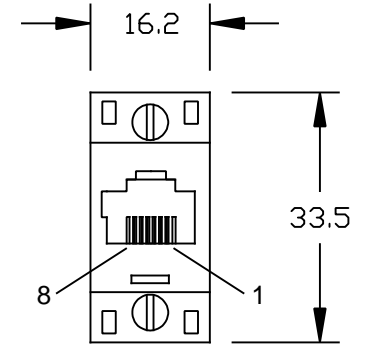
RJ45
