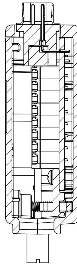
SECTION A-A
